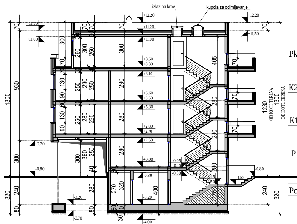
PRESJEK A-A
